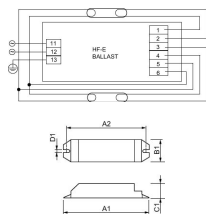
Technische Daten Philips HF-E 236 TL-D II 220-240V 50/60Hz für 2x36W
